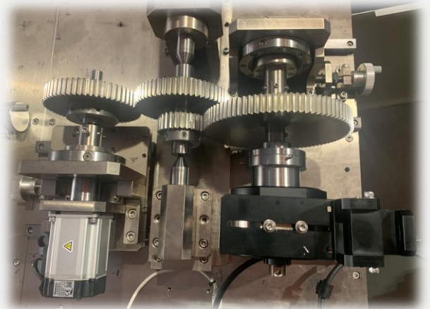
齒輪箱量測
